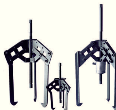
Стандартные механические съёмники SKF серии ТММР Удобные съёмники с двумя и тремя захватами
