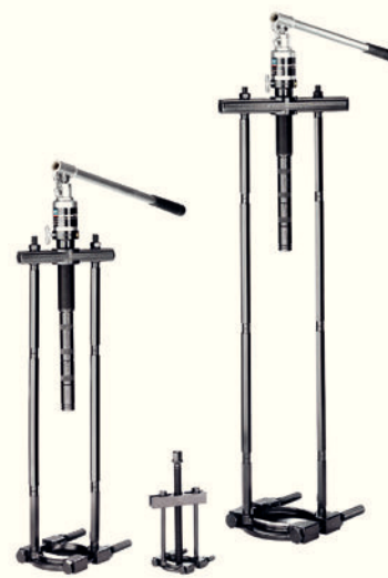
Обратные съёмники SKF серии ТМБС Е Лёгкий демонтаж подшипников даже в ограниченном пространстве
