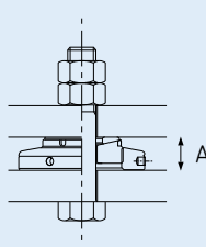
Низкопрофильные опоры SKF Vibracon
