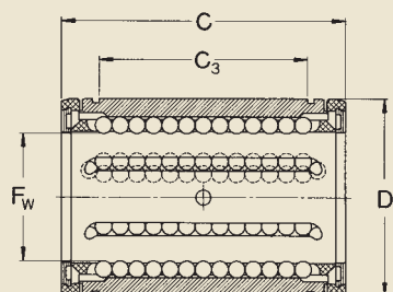
LBCR С защитными устройствами
