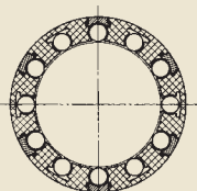
LBBR с двухкромочными уплотнениями
