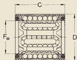
LBBR с двухкромочными уплотнениями
