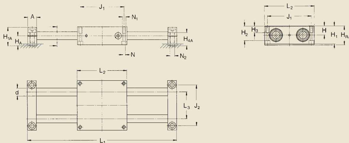
Конструкция LZBU ... A с закрытым подшипниковым узлом
