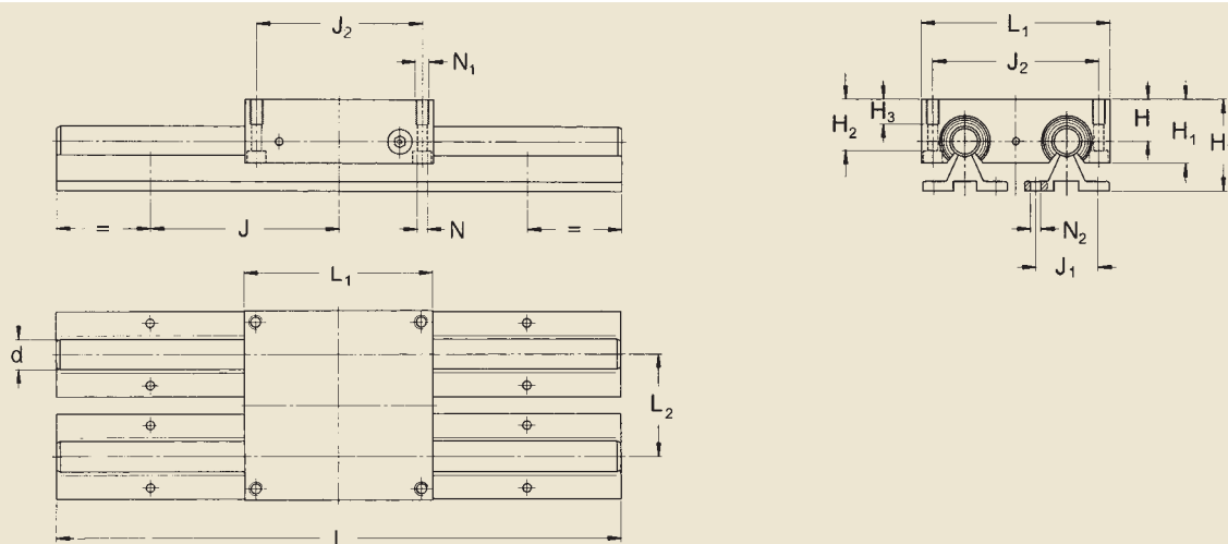
Конструкция LZAУ с открытым подшипниковым узлом типа LQCF
