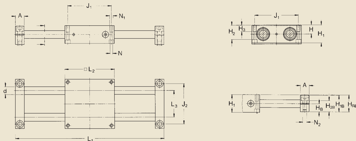
Конструкция LZBU ... В с закрытым подшипниковым узлом
