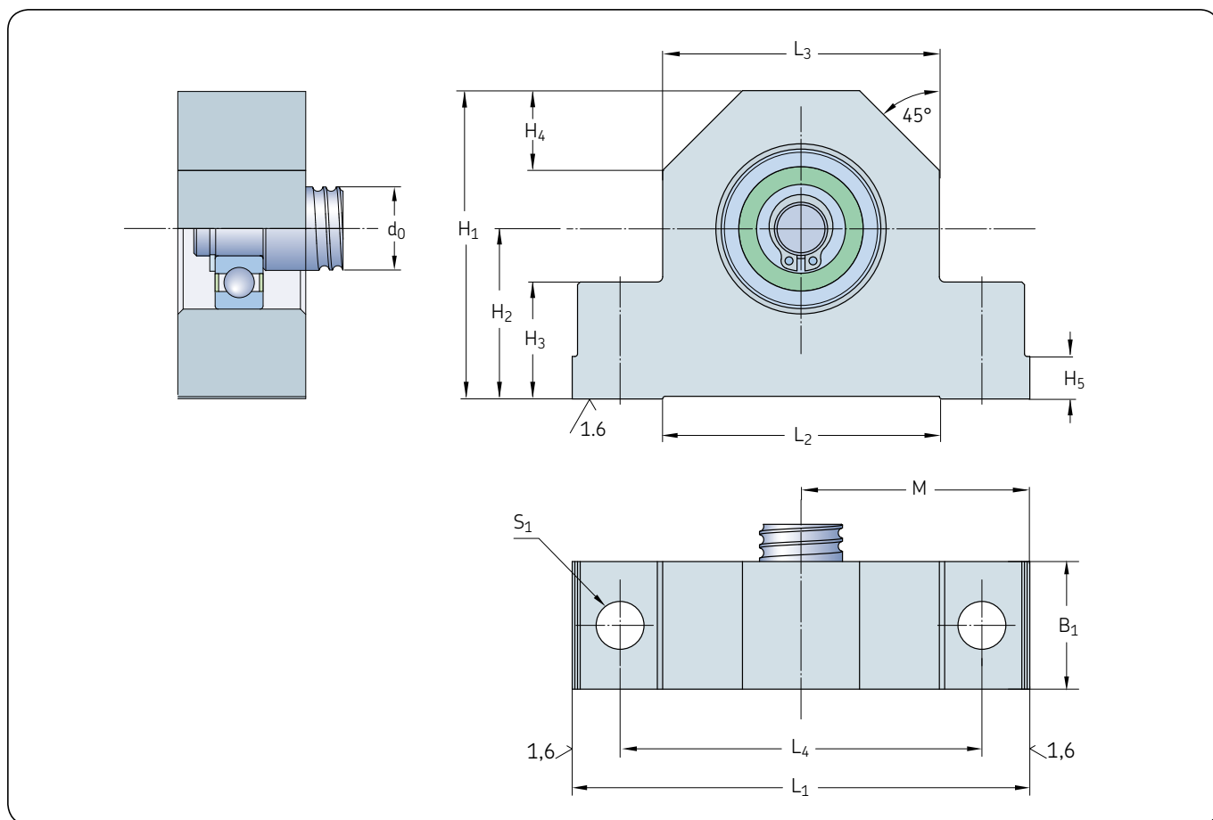
Винт Подшипниковая опора
