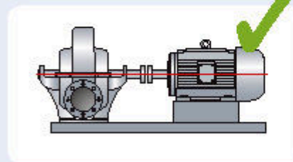
Точная соосность
