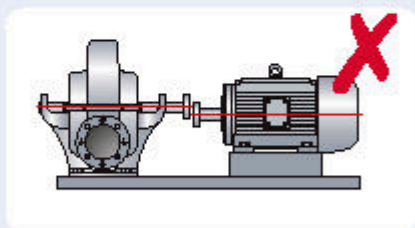
Параллельная несоосность (или сдвиг)
