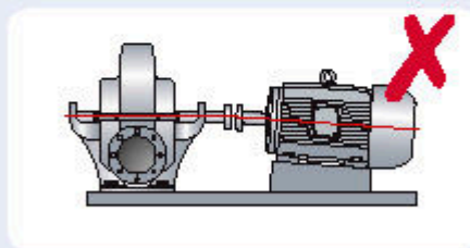
Угловая несоосность
