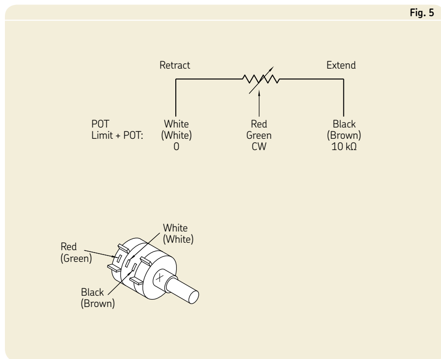
Potentiometer
