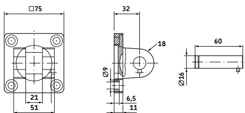
Swivel flange*
