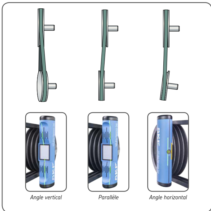
Figure 5 Résumé du désalignement
