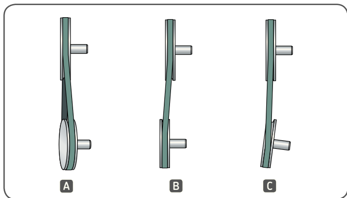
Figur 1 Olika typer av uppriktningsfel
