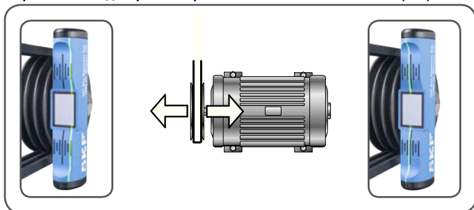
Figur 8 Parallellförsjutning upptäckt och efter korrigering
