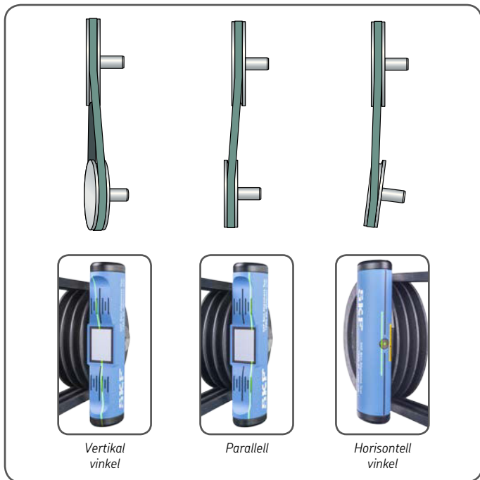
Figur 5 Sammanfattning riktfel
