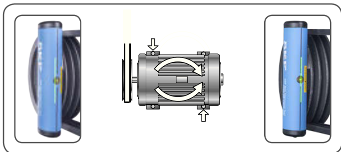
Аббидунг 7 Хоризонтален Винкелверсатз унд Аусрихтунг нах дер Корректур
